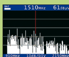
Kompleten SAT-spekter (910-2150 MHz);
