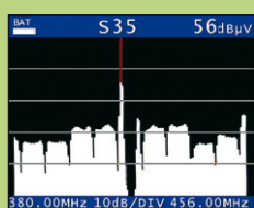
Spekter za analogni TV in 64 oz. 256 QAM;
